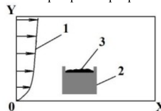
Рис. 2. Расчетная схема: 1 – профиль скорости ветра, 2 – полувагон, 3 – сыпучий груз
