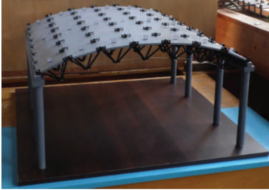
Рис. 2. Модель структурно-вантової циліндричної оболонки
