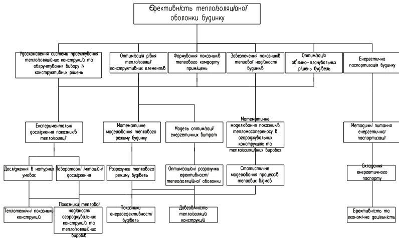
Рис.2 - Методичні положення рішення задачі забезпечення енергоефективності будинку
