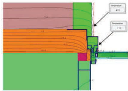
Рис. 5 – Температурне поле фактичного вузла примикання світлопрозорого стійкового-ригельного фасаду з холодним фальши фасадом до непрозорих зовнішніх стін
