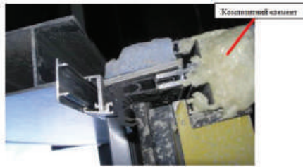
Рис. 4. Элемент жорсткості з композиту в стійки фальши фасаду
