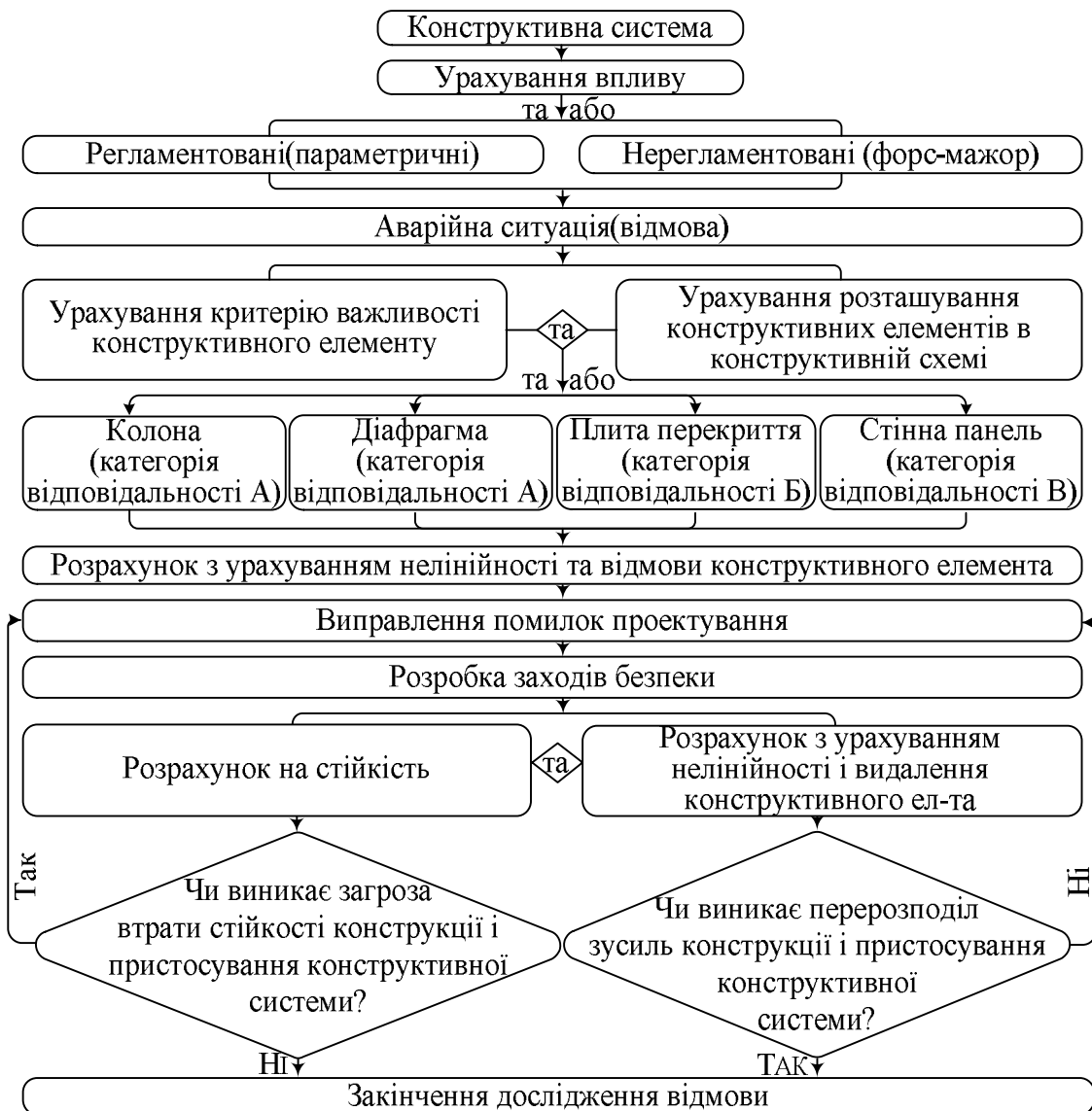
Рис. 3. Алгоритм причинно-наслідкового аналізу відмов для конструктивної системи / Algorithm for cause-and-effect analysis of refusals for structural system
