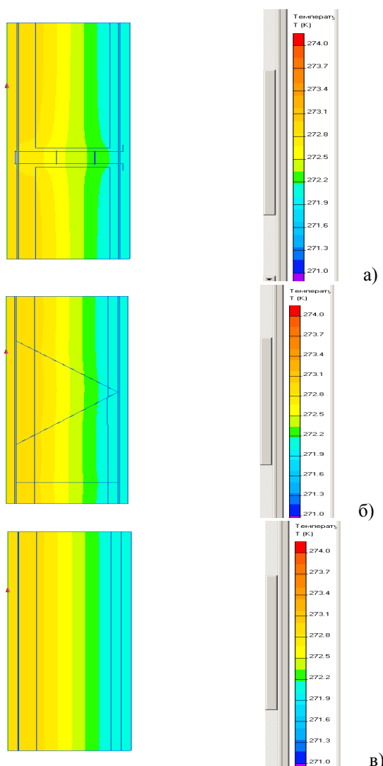
Рис. 1. Схема распределения температурных полей для трехслойной конструкции / The scheme of distribution of temperature fields in a three-layer structure:
