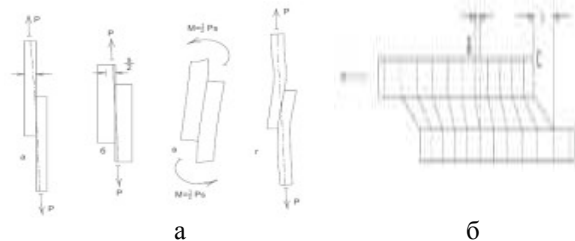
Рис. 4 Изгиб стены (а) и деформации сдвига в контактной зоне «кладка-покрытие» (б)
