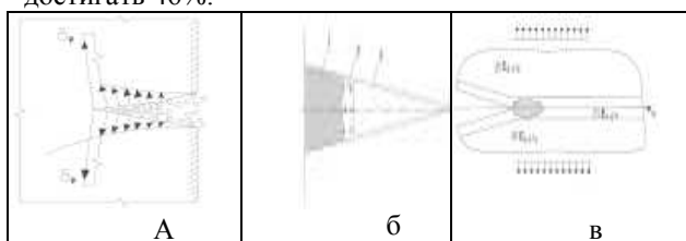
Рис. 8 Развитие магистральной трещины в контактной зоне под воздействием воды (а), и льда (б, в)
