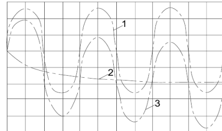
Рис.3 Температурные (1), усадочные (2) и суммарные деформации (3) и стеновой конструкции при эксплуатации
