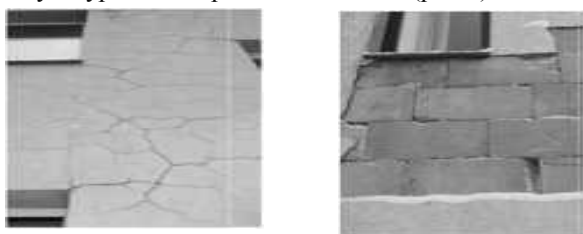
Рис. 9 Разрушение и отслоение штукатурного покрытия от газобетонной кладки
