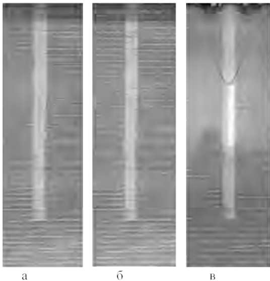
Рис. 5. Деформований стан основи при II серії випробувань: а – до випробування; б – 1-й етап (навантажувалась плита, нез'єднана з палею); в – 2-й етап (плита і палею з'єднанні між собою) / Fig. 5. Basis' strained state at the second series of tests: a - before the test; b - 1st stage (plate's fragment not connected with pile was loaded); c - 2nd stage (plate connected with pile)
