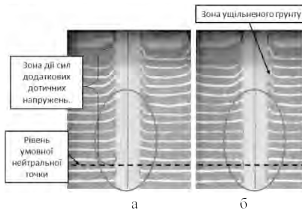
Рис. 9. Зображення впливу процесу почергового залучення елементів пального фундаменту до роботи на поведінку сил додаткового дотичного напруження і тертя вздовж бічної поверхні палі: а – навантажувалась плита, нез'єднана з палєю; б – не знімаючи прикладеного навантаження до плити, навантажувалась окремо палія / Fig. 9. Basis' strained state at the third series of tests: a – plate's fragment was loaded; b – without taking off the load applied to the plate, pile was loaded separately
