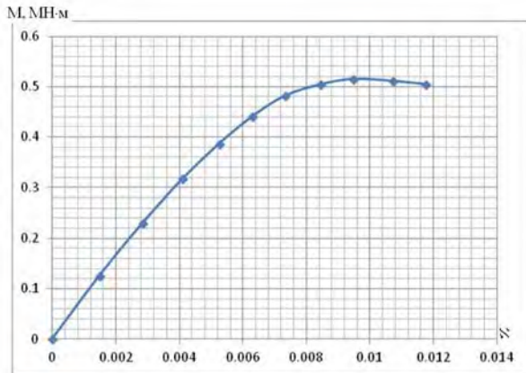
Рис. 4 - Діаграма стану перерізу залізобетонної балки/
