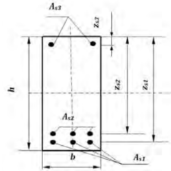
Рис.3. Переріз балки/ Beam section
