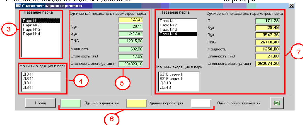
Рис. 3. Интерфейс сравнения параметров выбранных парков скреперов: 3-название парка; 4-Машины входящие в парк; 5-суммарный показатель параметров парков скреперов; 6-эффективное цветное выделение параметров парка; 7- техническая характеристика выбранного парка.
