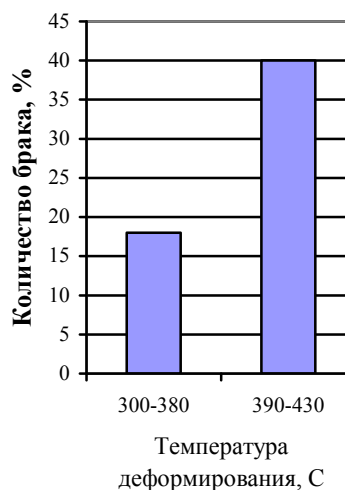
Рис. 2. Влияние температуры деформации на количество брака расслоений в штамповках сплава В95
