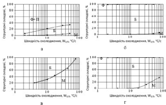
Рис. 2. Діаграми структурних перетворень аустеніту на ділянці перегріву металу ЗТВ мікролегованих сталей типу: а – 06ГБД; б – 06Г2Б; в – 09Г2СЮч; з – 10Г2ФБ
