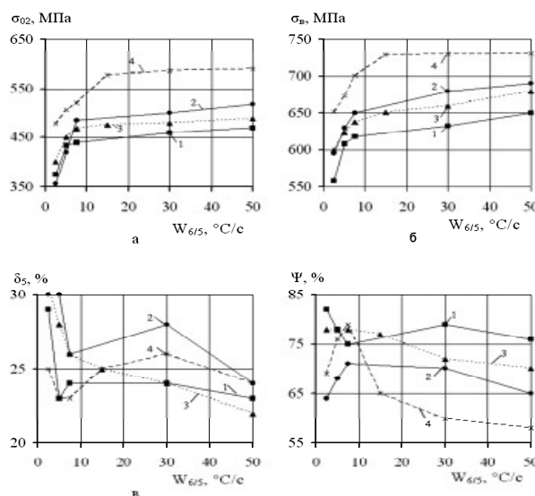
Рис. 7. Вплив швидкості охолодження W_{6/5} на показники границі текучості (а), границі міцності (б), відносного подовження (в) та відносного звуження (г) металу ЗТВ сталей: 06ГБД (1), 09Г2СЮч (2), 06Г2Б (3), 10Г2ФБ (4)
