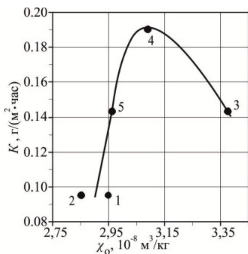
Рис. 2. Зависимость скорости коррозии K [5] от удельной магнитной восприимчивости \chi_0 аустенита исследуемого сплава 06ХН28МДТ (№ плавки 1...5) / Dependences of the corrosion rate K [5] on the specific magnetic susceptibility \chi_0 austenite of the investigated alloy 06HN28MDT (number of heats 1 ... 5)
