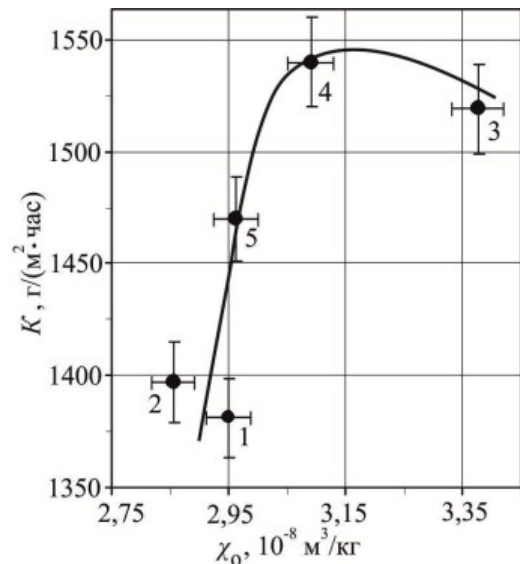
Рис. 1. Зависимость скорости коррозии K от удельной магнитной восприимчивости \chi_0 аустенита исследуемого сплава 06ХН28МДТ (№ плавов 1...5) / Dependences of the corrosion rate K on the specific magnetic susceptibility \chi_0 austenite of the investigated alloy 06HN28MDT (number of heats 1...5)
