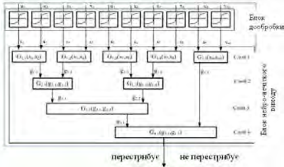
Рис. 2. Алгоритм каскадної нейро-нечіткої мережі для побудови моделі успішності стрибка
