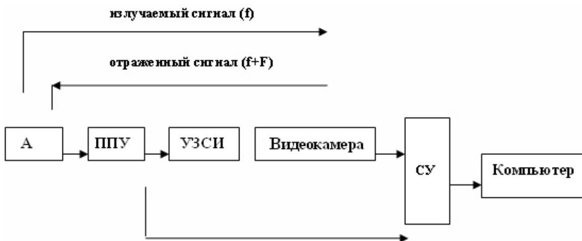
Рис. 2. Структурная схема радиолокационной установки для получения звуковой срочной информации о скорости разгона легкоатлетических снарядов
