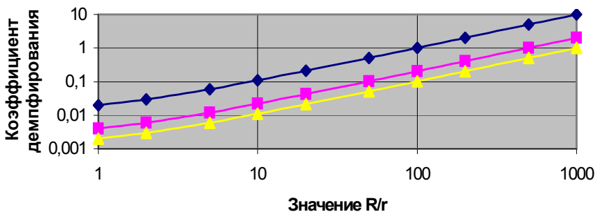
Рис. 4. Зависимость коэффициента демпфирования от R/r и Q
