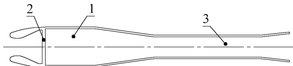
Рис. 1. Схема ПуВРД
