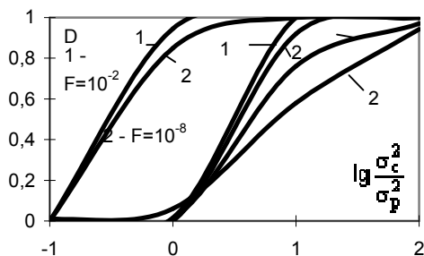
Рис. 8. Характеристики обнаружения
