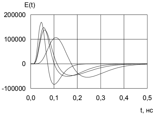
Рис. 7. Уширение СШП сигнала
