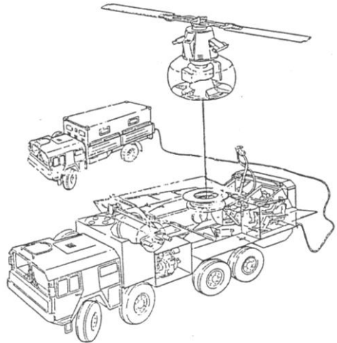
Рис. 1. Подвижный вариант длинновыдвижной тросовой системы
