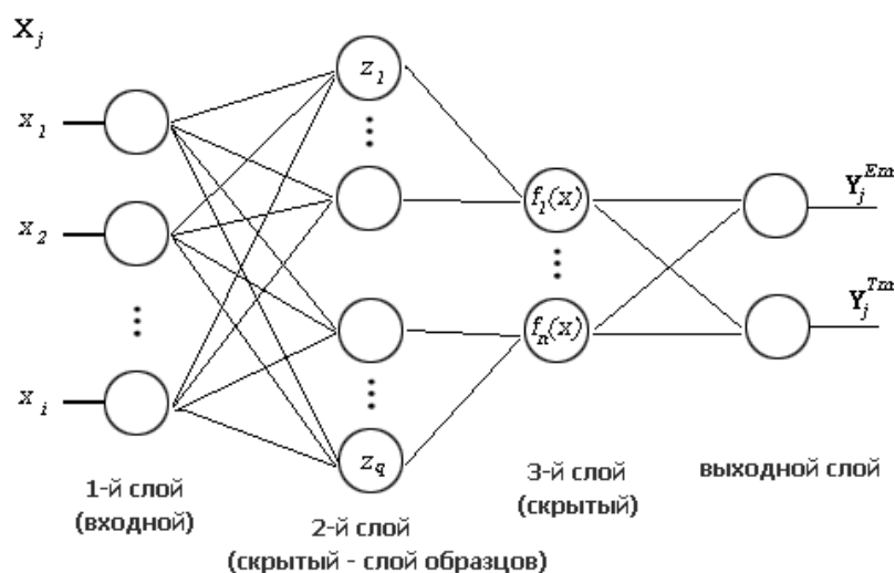
Рис. 5. Архитектура PNN-сети
