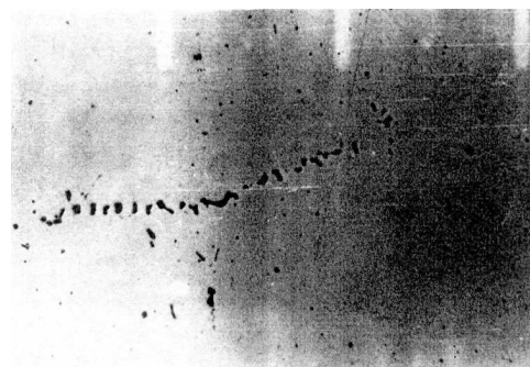
Рис. 9. Неметаллические включения в ободу колеса № 81-298480-8-425580 (М-188) (увеличено в 100 раз)
