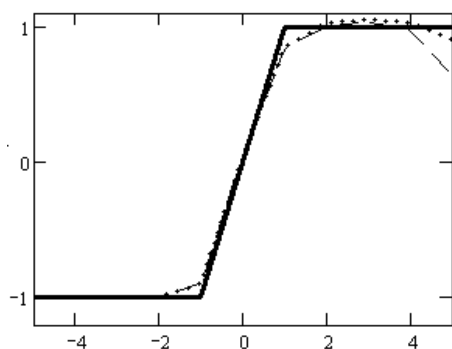
Рис. 5. Шаговая функция
