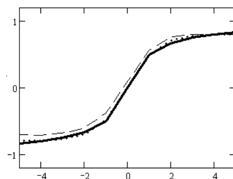
Рис. 4. Сигмоидальная функция
