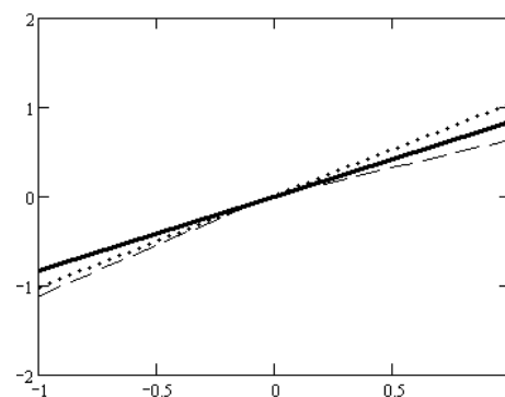
Рис. 3. Синусоидальная функция
