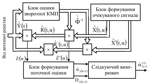
Рис. 2. Структурна схема вимірювача напрямку приходу сигналу при формуванні поточної оцінки по |\dot{Z}(\alpha)|
