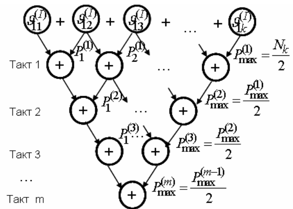
Рис. 1. Алгоритм сдваивания
