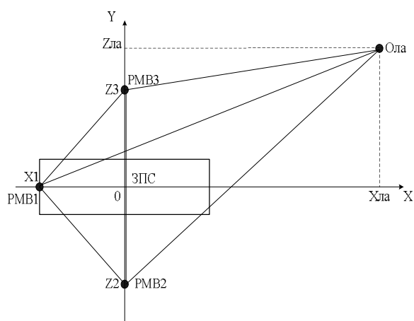
Рис. 2. Варіант розміщення РТЗ, який пропонується при посадці на необладнаний аеродром
