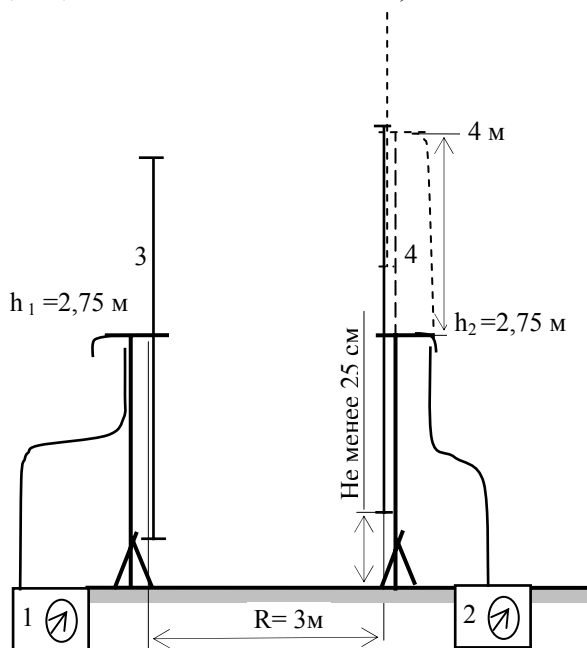
Рис. 1. Схема измерения затухания площадки при вертикальной поляризации:
