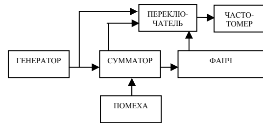
Рис. 1. Структурная схема
