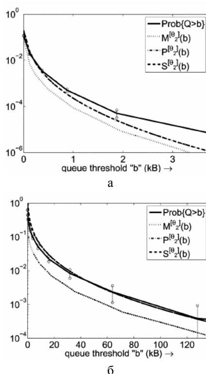
Рис. 1. Сравнение аппроксимаций максимума, произведения и суммы с P\{Q_\infty > b\} для трафика ФГШ с параметром H=0,8 , пропускной способностью канала 10 Мб/с и \sigma = 8 \times 10^5 бит: а – 30% использования; б – 80% использования
