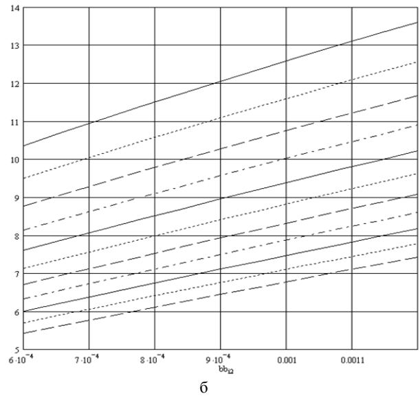
Рис. 6. Зависимость угла сдвига фаз между гармоническими колебаниями напряжения и тока от поляризационной емкости аккумулятора (а – f = 0,1 Гц; б – f = 1 Гц)
