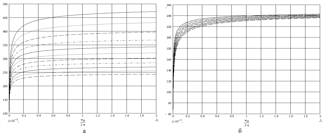
Рис. 4. Влияние частоты входного сигнала на амплитуду выходного сигнала (а – при постоянной поляризационной емкости; б – при постоянном внутреннем сопротивлении)
