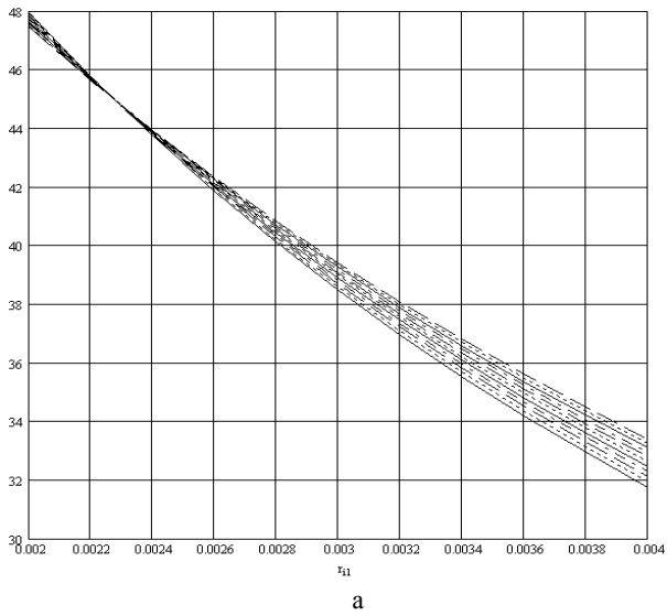
Рис. 5. Зависимость угла сдвига фаз между гармоническими колебаниями напряжения и тока от омического сопротивления аккумулятора (а – f = 0,1 Гц; б – f = 1 Гц)
