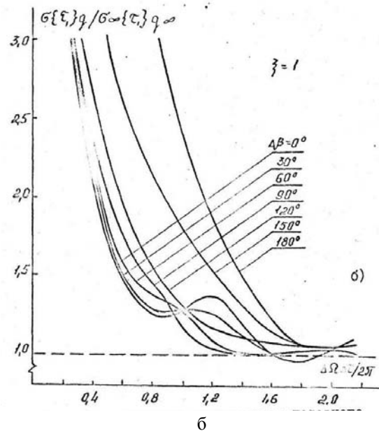
Рис. 1. Зависимость нормированной среднеквадратической ошибки измерения запаздывания полезного сигнала от степени перекрытия ( \Delta\Omega\Delta\tau/2\pi ) полезного и мешающего сигналов, разности фаз ( \Delta\beta ) между ними и амплитуды ( \zeta ) мешающего сигнала (для прямоугольной формы спектра зондирующего сигнала)
