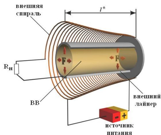
Рис. 1. Спиральный ВМГ
