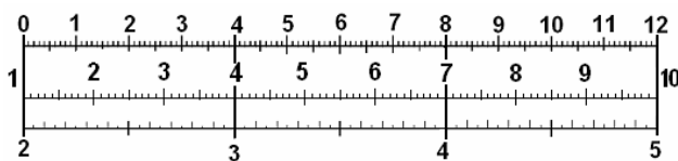
Рис. 4. Лінійаризована залежність оцінок чотирьох-, десяти- та дванадцятибальної шкал
