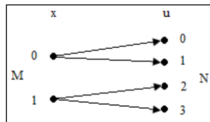
Рис. 7. Отображение f(x) = u
