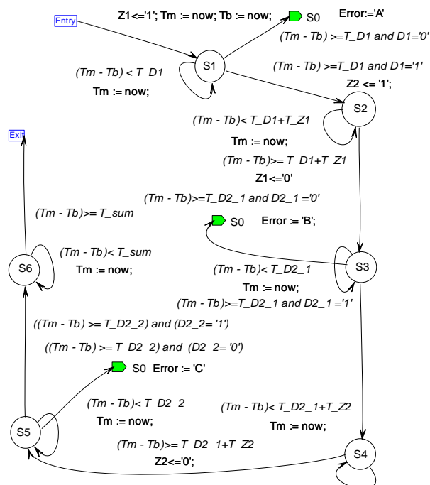
Рис. 2 Иерархический граф нижнего уровня цифрового автомата
