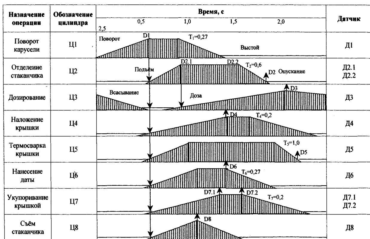
Рис. 1 Циклограмма работы исполнительных механизмов
