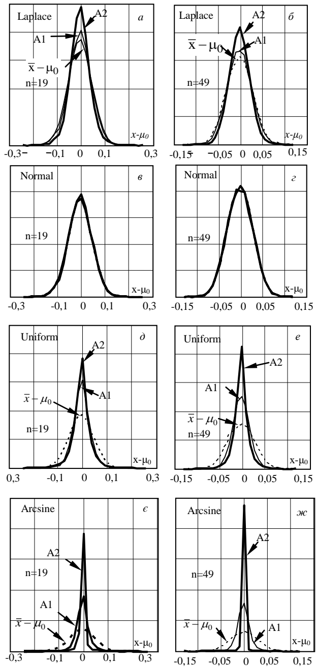
Рис. 5. Гістограми похибок визначення параметру положення
