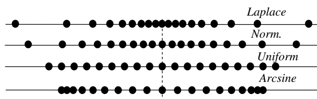
Рис. 1. 4 набори зразкових спостережень ( n = 19 )
