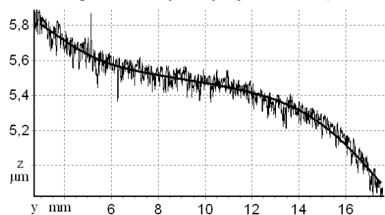
Рис. 6. Профилограмма, описывающая случайную функцию Z_3(y) верхней поверхности покрытия в пределах от y_3 до y_4 (увеличение)
