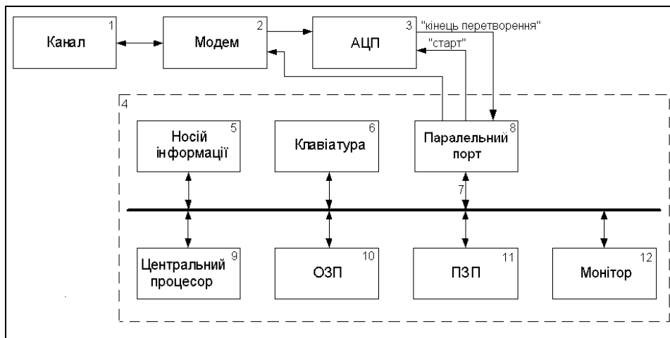
Рис. 1. Схема пристрою для обміну інформацією
