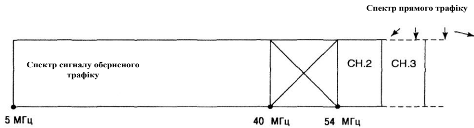
Рис. 7. Низькочастотна частина спектру радіосигналу в сервісі КТБ.
