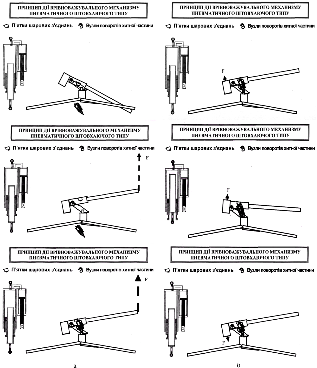
Рис. 3. Динамічна інтерактивна демонстрація принципу дії врівноважувального механізму гармати: а – ствол гармати невірноважений і вимагає значних сил для переміщень; б – ствол гармати врівноважений і вимагає малих зусиль для наведення
