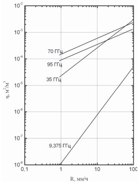
Рис. 3. Усредненные \eta , полученные в BRL для четырех частот микроволнового диапазона
