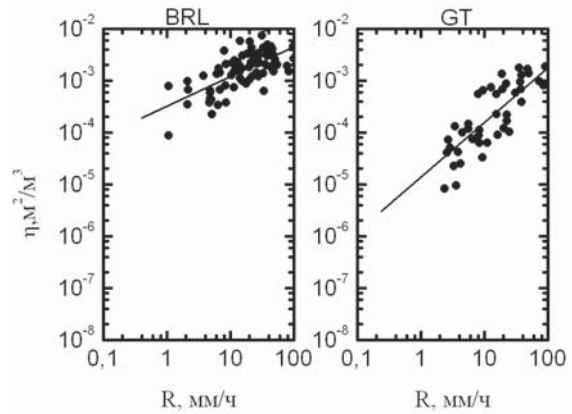
Рис. 5. Сопоставление пиковых \eta , полученных в BRL и GT на частоте 95 ГГц
