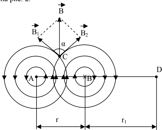
Рис. 2. Силві лінії магнітного поля двопровідної лінії
