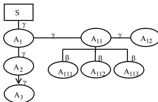
Рис. 3. Приклад логічної моделі інтегральної оцінки фактору S
