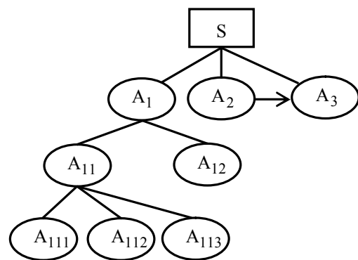
Рис. 1. Приклад ієрархічної системи показників, що визначають інтегральну оцінку здатності сторони вести збройну боротьбу
