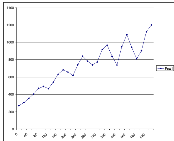
Рис. 2. Замеры температуры для z = 1/2
