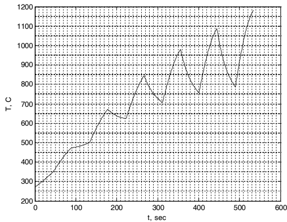
Рис. 1. Расчетное температурное распределение для z = 1/2
