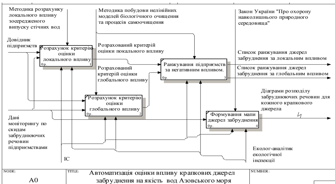
Рис. 1. Контексна діаграма
