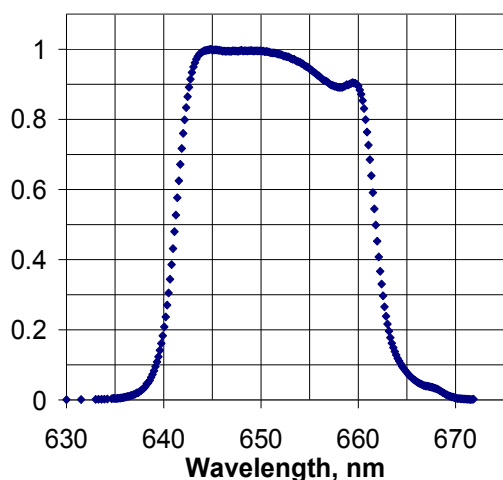
Рис. 6. Спектральна чутливість TSP-2
