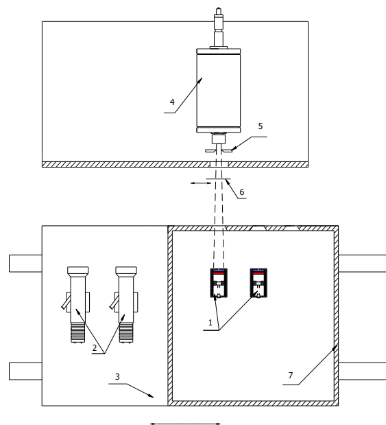
Рис. 8. Установка для калібрівки радіаційних термометрів по фільтровим радіометрам з допомогою чорного тіла
