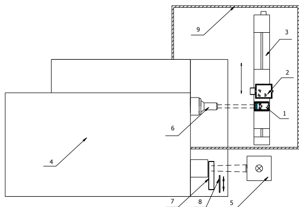
Рис. 5. Спектральний компаратор
