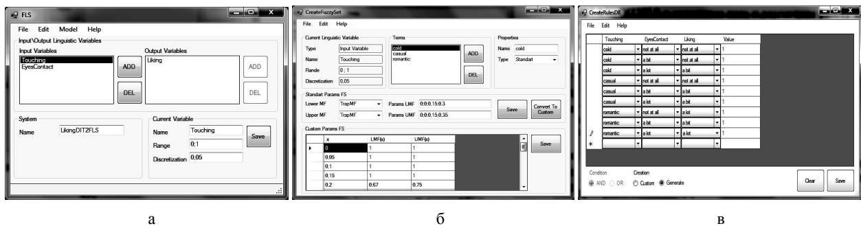
Рис. 2. Интерфейс DIT2FLS Toolbox: а – редактор лингвистических переменных; б – редактор функций принадлежности лингвистических переменных; в – редактор базы правил
