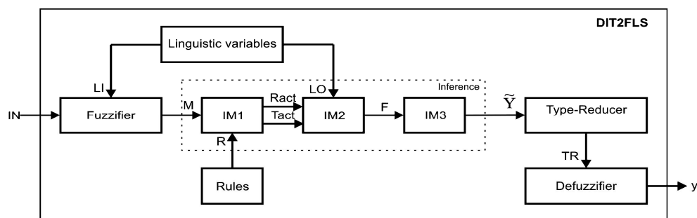
Рис. 1. Структура DIT2FLS
