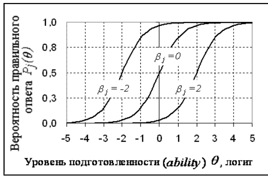
Рис. 2. Характеристические кривые заданий (ICC)
