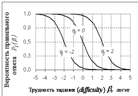
Рис. 3. Характеристические кривые испытуемых (PCC)
