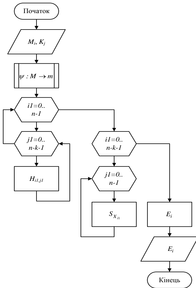
Рис. 1. Алгоритм формування криптограм
