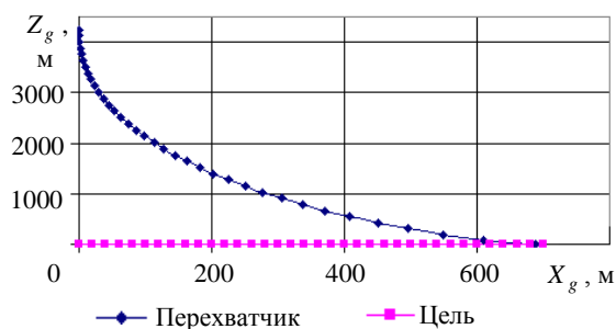
Рис. 1. Траектории истребителя и цели при начальной дальности до цели D_0 = 4\ 250\ \text{м}
