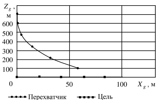
Рис. 3. Траектории цели и перехватчика при начальной дальности до цели D_0 = 711\ \text{м}
