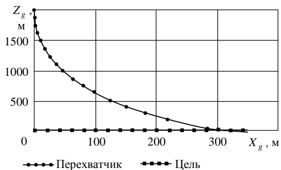
Рис. 2. Траектории цели и перехватчика при начальной дальности до цели D_0 = 2\ 000\ \text{м}
