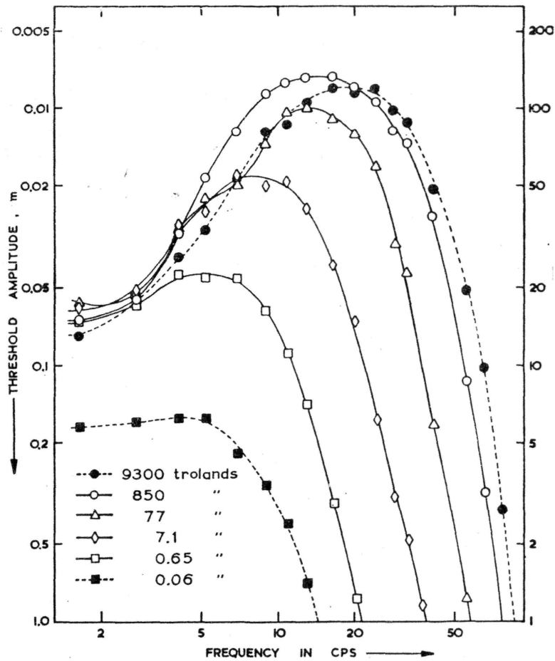
Рис. 4. Залежність обмірюваної чутливості амплітуди модуляції, що виявляється мінімально, від частоти для шести різних рівнів фотопічної адаптації до білого світла (спостерігач ДНК)
